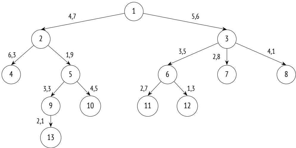
Рис. 2.11. Иерархические данные
