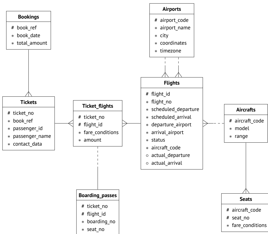
Рис. 2.6.3. Схема демонстрационной базы данных
