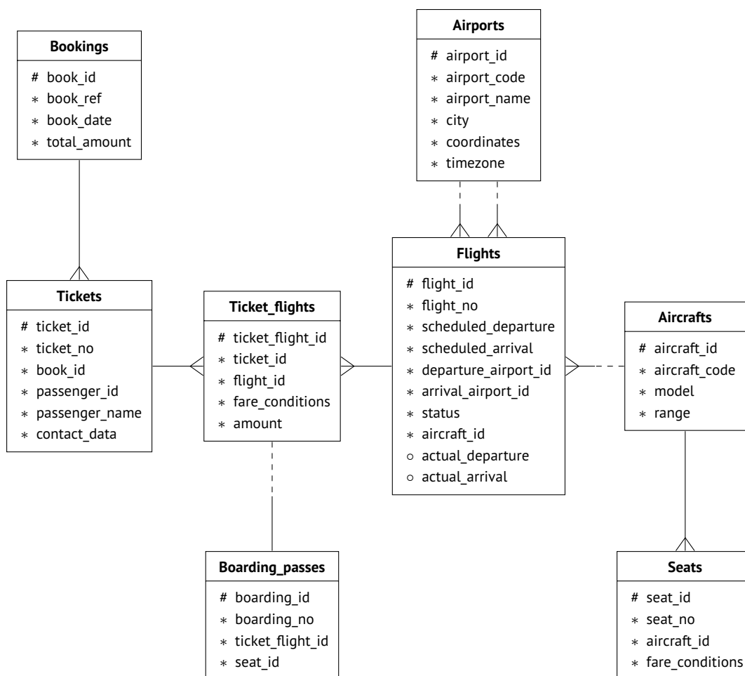
Рис. 2.6.2. Фрагмент схемы БД для хранения авиабилетов с суррогатными ключами
